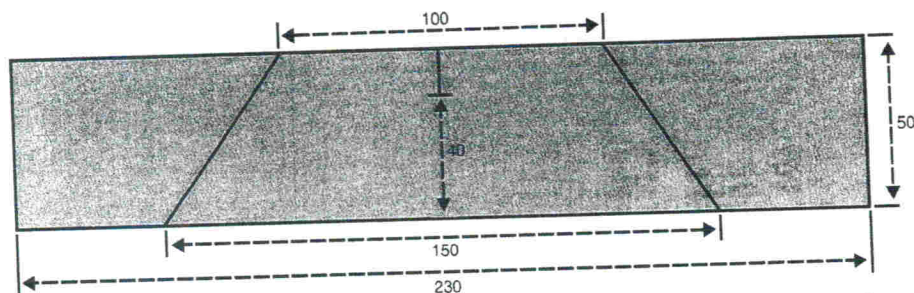
Figura 2 – Corpo de prova trapezoidal (medidas em mm)
